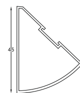
SCP - 72 Corner Pipe Size : 6 mtr. Finish : Black Matt
