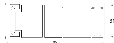
SCP - 131 Door Frame Profile Size : 3 mtr. Finish : Aluminium
